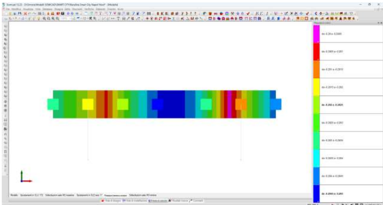
Figura 1 Pressioni massime in fondazione Fermata bus
